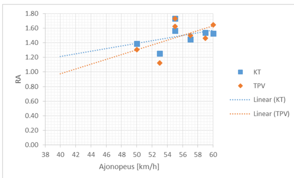
Kuva 29. 84 t HCT-puutavarayhdistelmän ajoneuvoyksiköiden RA-arvot ISO 3888-1 standardin mukaisessa kaksoiskaistanvaihtokokeessa määritettynä ajoneuvoyksiköiden sivuttaiskiirtyvyyksistä.
