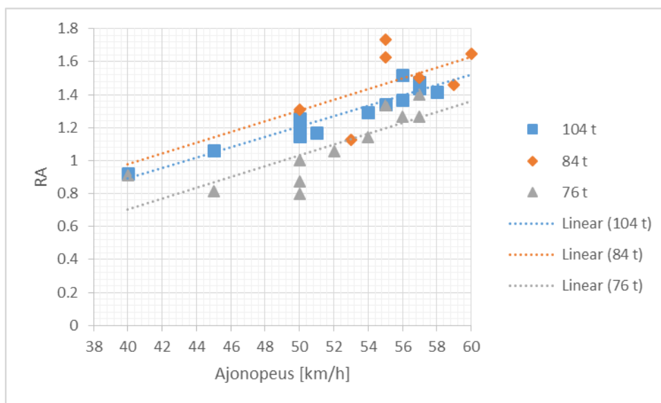
Kuva 33. Kuormattujen ajoneuvoyhdistelmien RA-arvot ISO 3888-1 standardin mukaisessa kaksoiskaistanvaihtokokeessa sivuttaiskiihtyvyydestä määritettynä.
