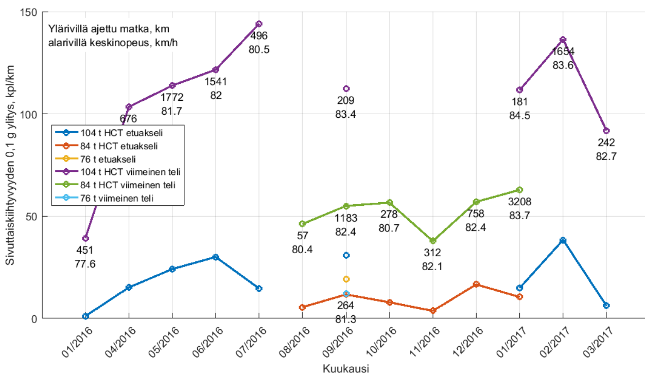
Kuva 16. Kuormattujen yhdistelmien 0,1 g sivuttaiskiintiyyden ylitys, vain yli 70 km/h ajonopeus mukaan luettuna.
