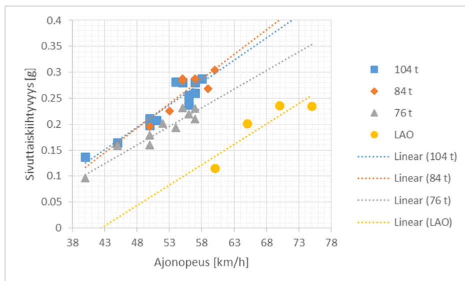
Kuva 34. Ajoneuvoyhdistelmien viimeisten akselien suurimmat sivuttaiskiikityvydet ISO 3888-1 standardin mukaisessa kaksoiskaistanvaihtokokeessa.
