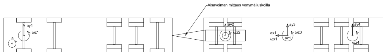
Kuva 4. Mittausjärjestelmä P&A Trans Oy:n 84 t HCT-yhdistelmässä.
