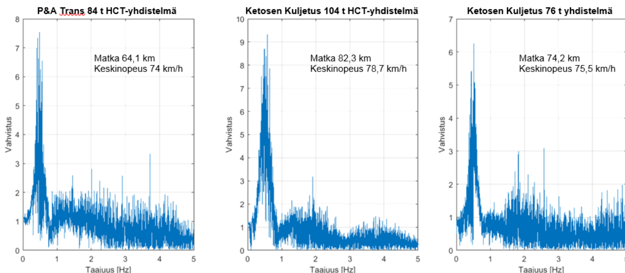
Kuva 19. Tutkimusyhdistelmien sivuttaiskiivyyden vahvistuminen etuakselilta täysperävaunun takatelille, syyskuu 2016, valtatie 4.
