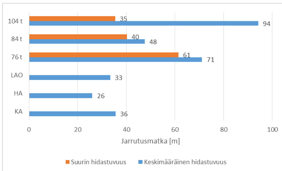
Kuva 35. Ajoneuvojen sekä ajoneuvoyhdistelmien laskennalliset jarrutusmatkat määritettynä keskimääräiselle sekä suurimmalle hidastuvuudelle nopeudesta 80 km/h.
