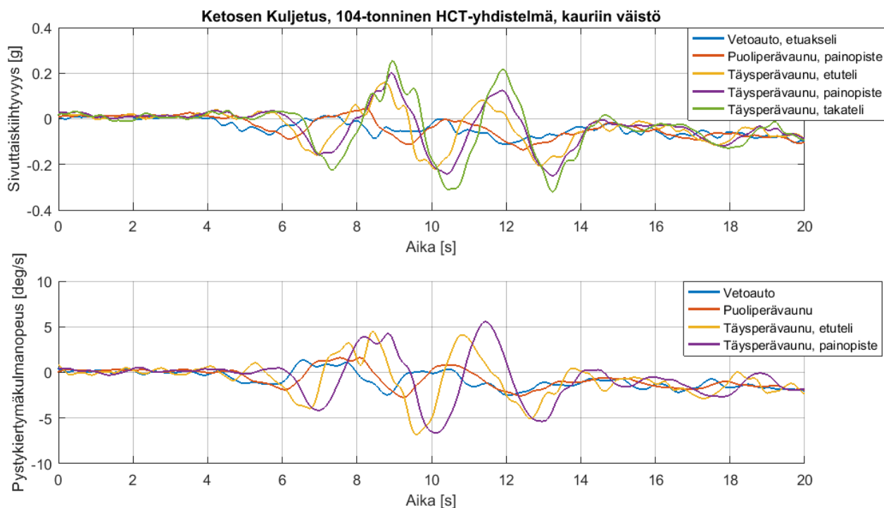
Kuva 22. Kauriin väistö Ketosen Kuljetuksen HCT-yhdistelmällä 25.5.2016.
