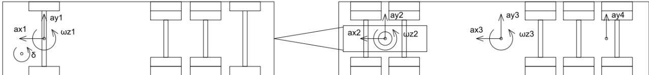
Kuva 7. Vertailuyhdistelmän anturointi.
