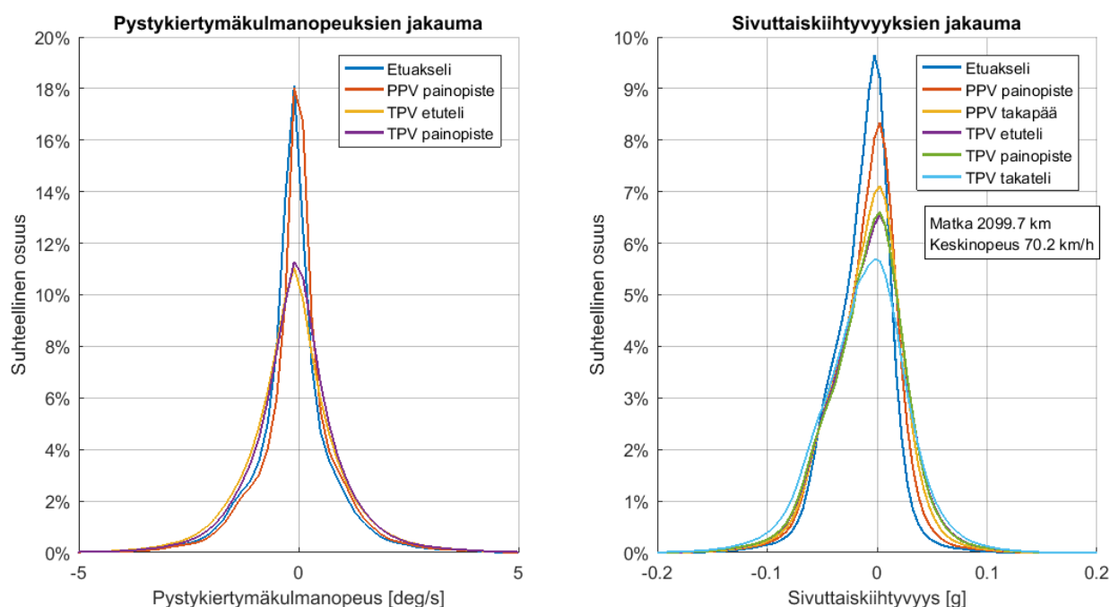
Kuva 12. Ketosen Kuljetus, 104 t HCT-yhdistelmä, liiketilasuureiden jakaumat, toukokuu 2016.
