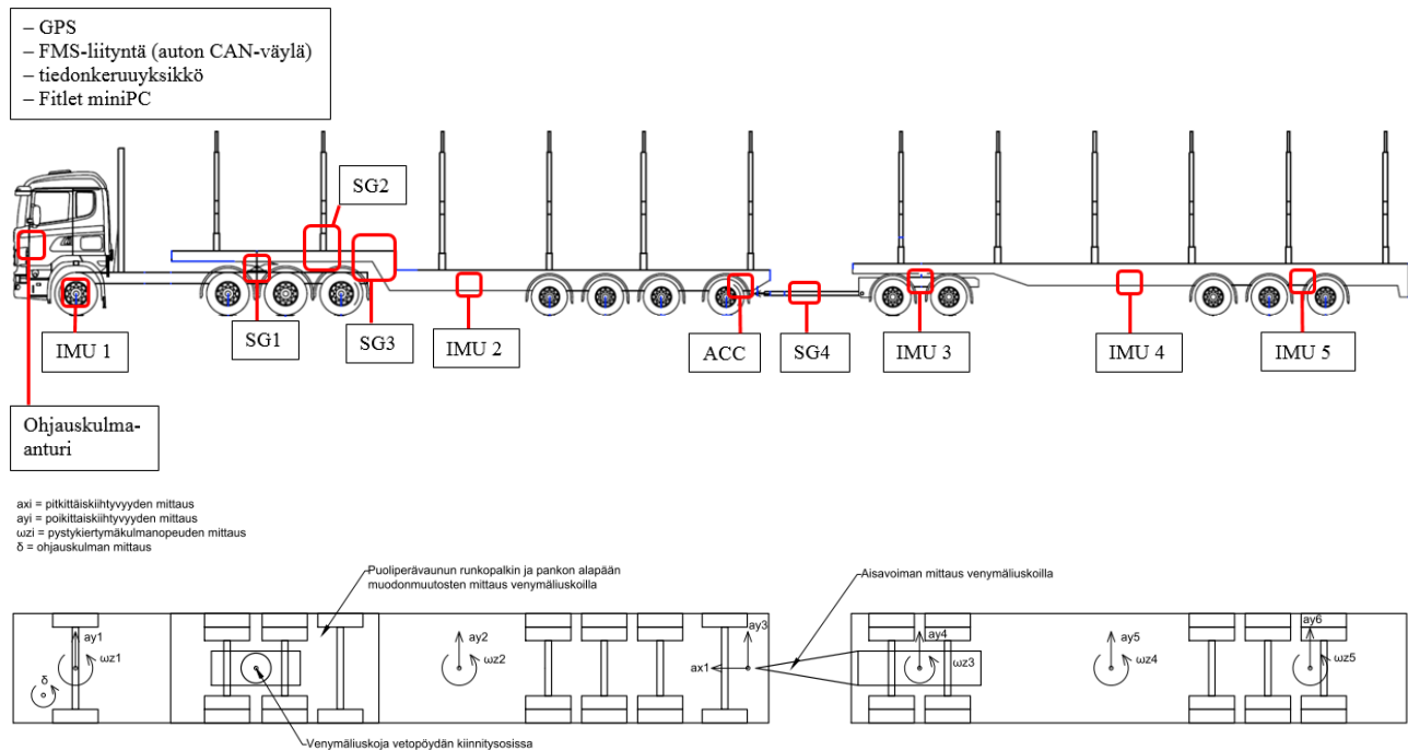
Kuva 3. Mittausjärjestelmä Ketosen Kuljetus Oy:n 104 t HCT-yhdistelmässä.
