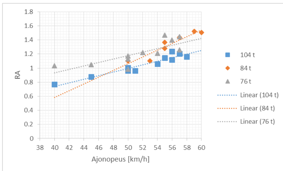
Kuva 32. Kuormattujen ajoneuvoyhdistelmien RA-arvot ISO 3888-1 standardin mukaisessa kaksoiskaistanvaihtokokeessa pystykiertymäkulmanopeudesta määritettynä.
