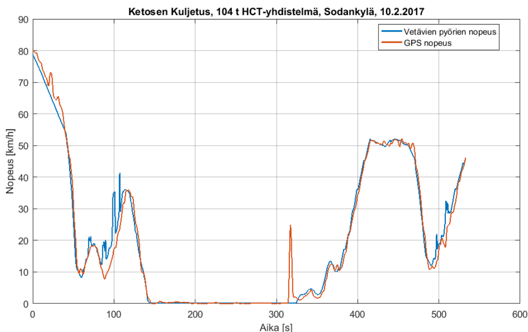
Kuva 9. Ketosen Kuljetuksen HCT-yhdistelmän pyörä- ja GPS-nopeudet Sodankylän taajamassa valtatiellä 4 10.2.2017.
