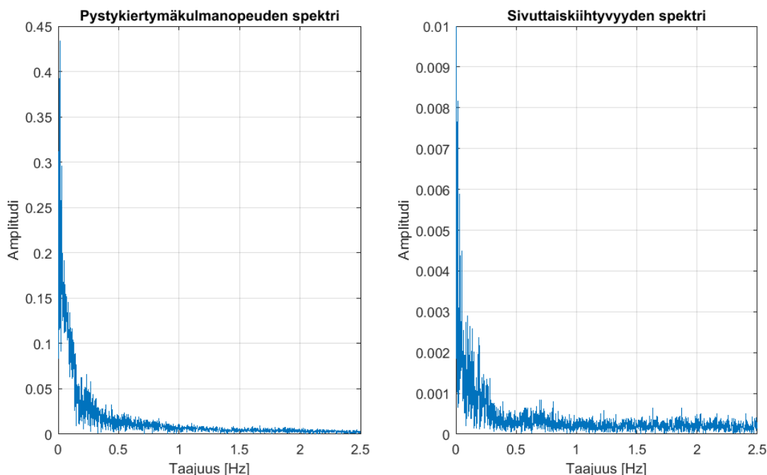
Kuva 20. P&A Trans Oy:n HCT-yhdistelmän etuakselilta mitattujen herätteiden taajuusspektrit 20.9.2016.
