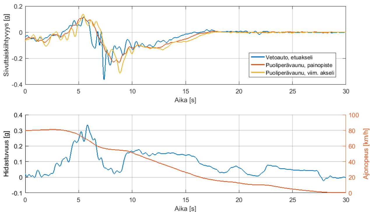
Kuva 23. Henkilöauton väistö Ketosen Kuljetuksen HCT-yhdistelmällä 5.7.2017.
