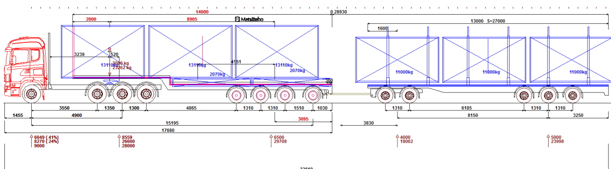
Kuva 1. Ketosen Kuljetus Oy:n 104 t HCT-yhdistelmä.
