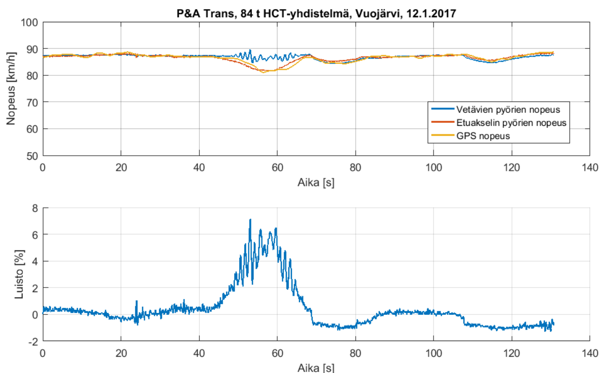
Kuva 10. P&A Trans, 84 t HCT-yhdistelmä valtatiellä 4 Vuojärvellä 12.1.2017, luistoa ajon aikana.
