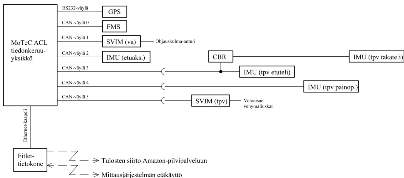
Kuva 6. Mittausjärjestelmän kytkennät P&A Trans Oy:n HCT-yhdistelmässä.
