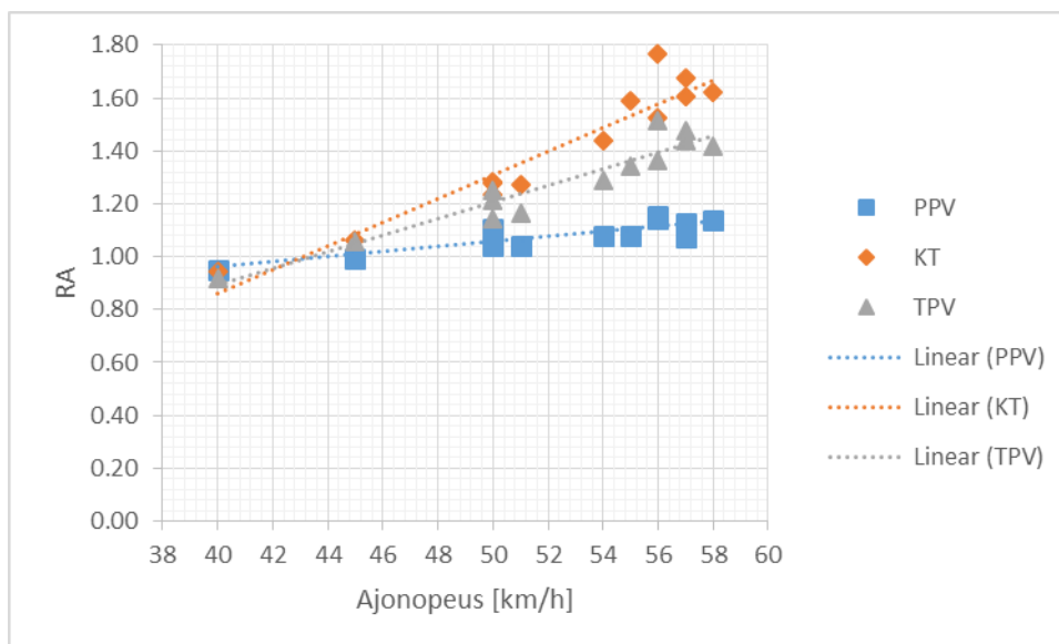
Kuva 27. 104 t HCT-puutavarayhdistelmän ajoneuvoyksiköiden RA-arvot ISO 3888-1 standardin mukaisessa kaksoiskaistanvaihtokokeessa määritettynä ajoneuvoyksiköiden sivuttaiskiihtyvyyksistä.
