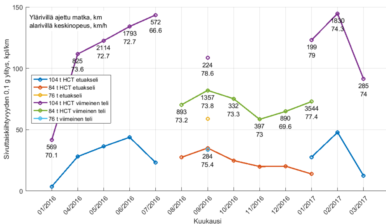
Kuva 15. Kuormattujen yhdistelmien 0,1 g sivuttaiskiintiyyden ylitys, kaikki ajonopeudet mukaan luettuna.
