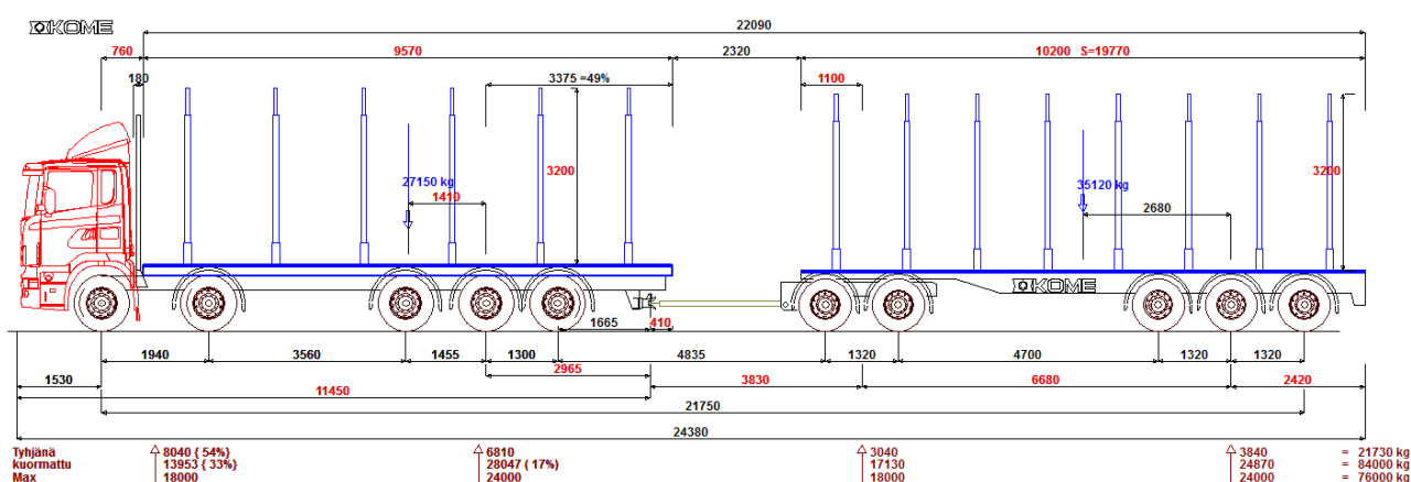
Kuva 2. P&A Trans Oy:n 84 t HCT-yhdistelmä.
